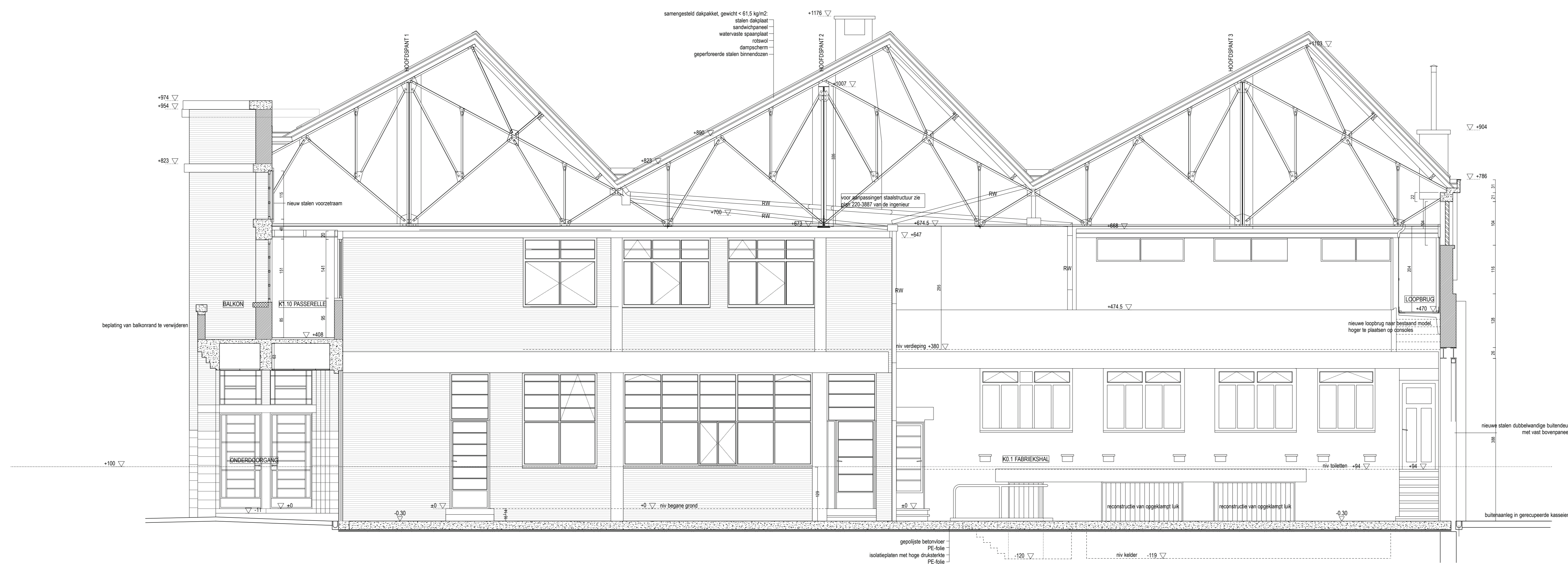
DOORSNEDE 7 MET ZICHT OP BINNENGEVEL
