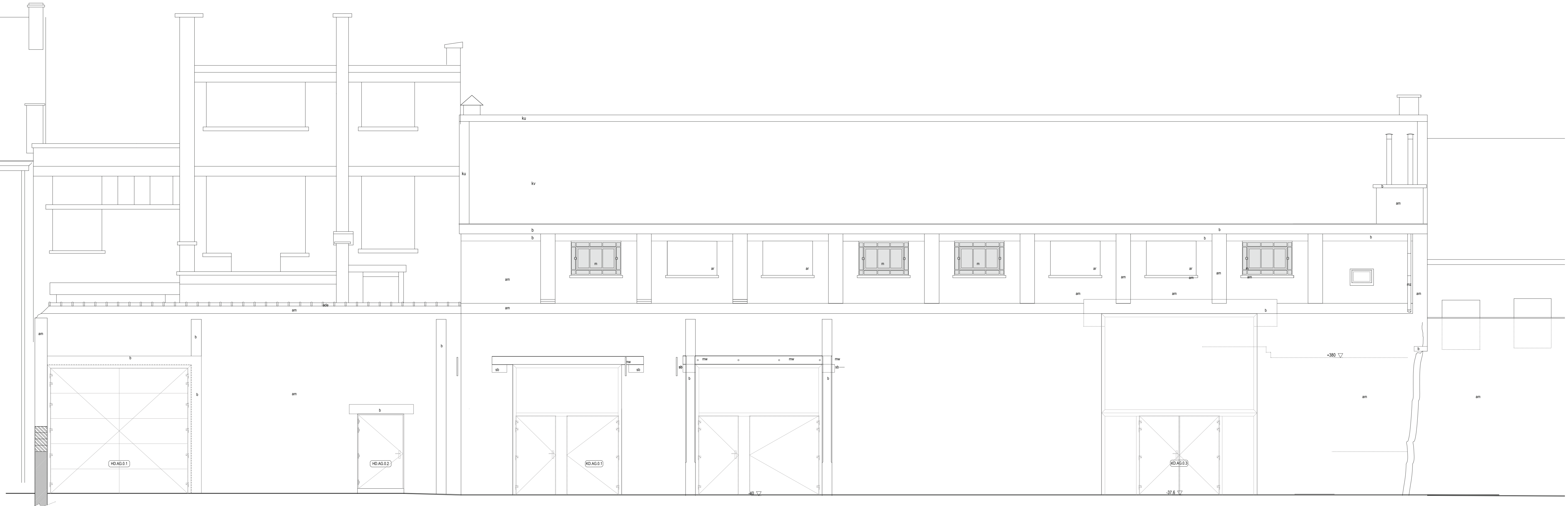
ACHTERGEVEL HUIS HOSTE
